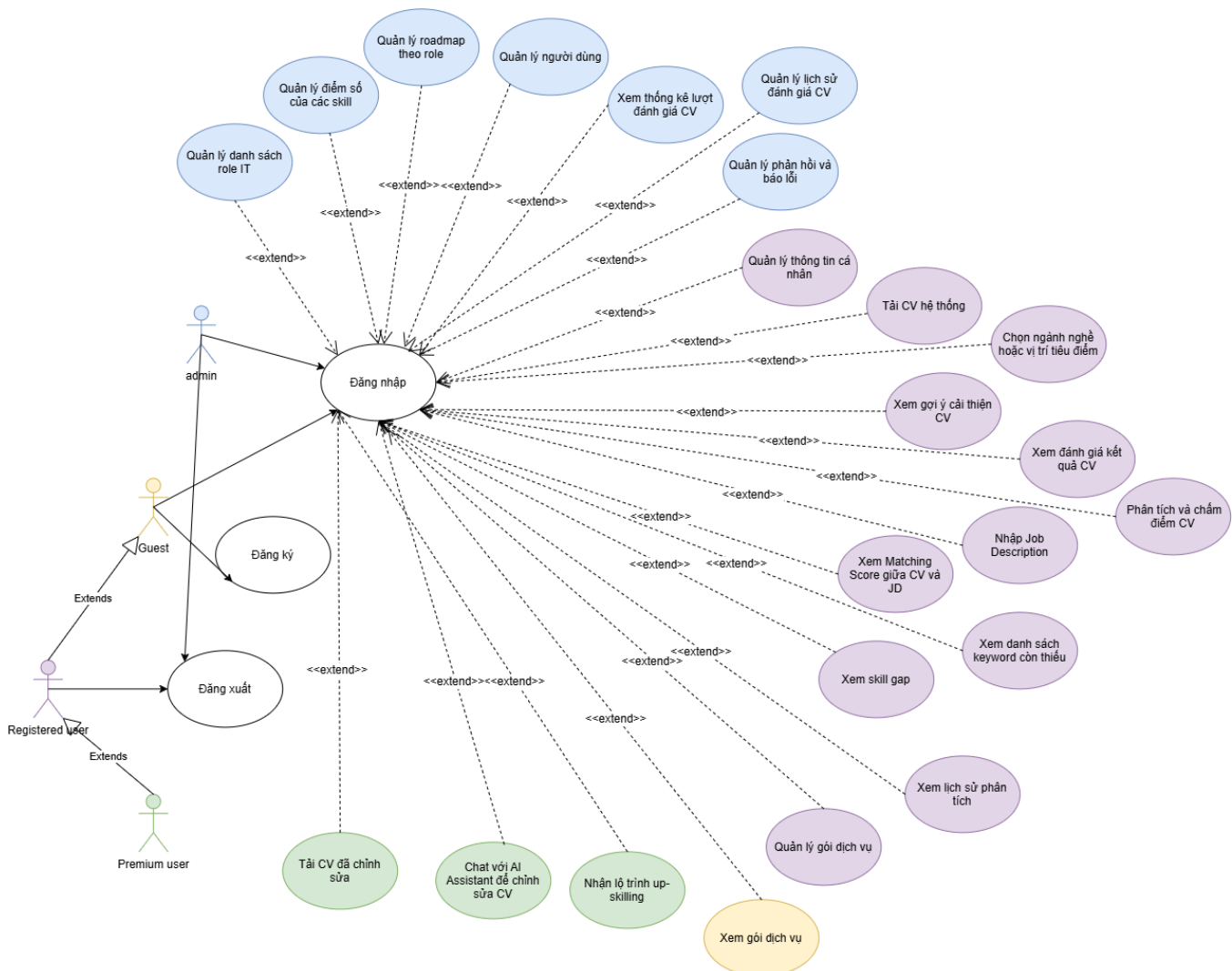
Hình 3: Sơ đồ Use Case tổng thể của hệ thống SmartCV Advisor
