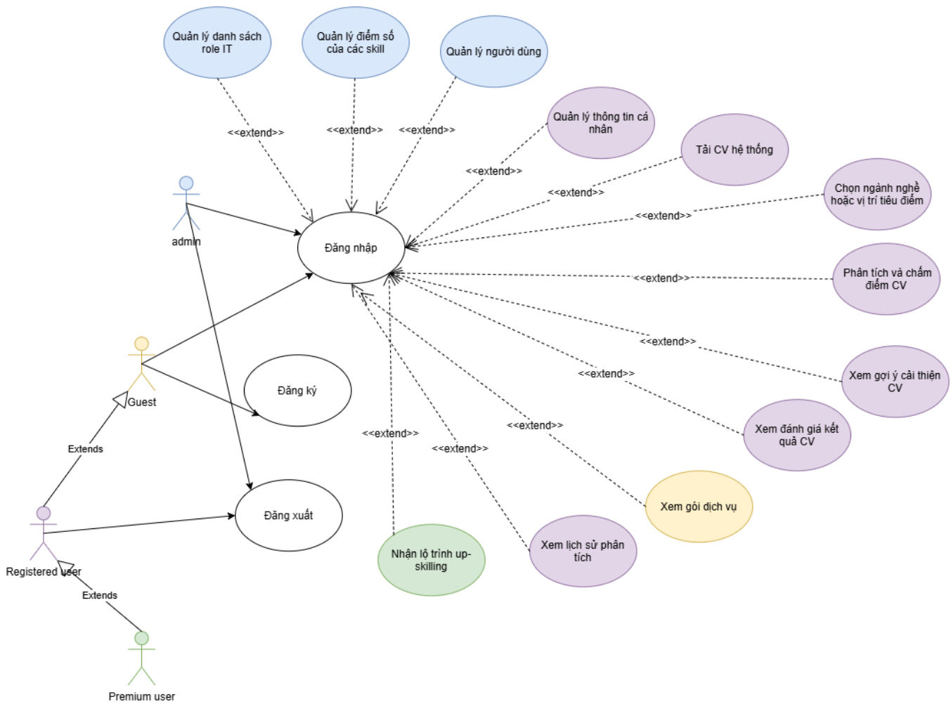
Hình 4: Sơ đồ Use Case của phiên bản MVP SmartCV Advisor
